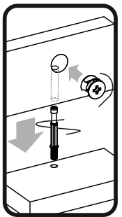
схема монтажа эксцентриковой стяжки
