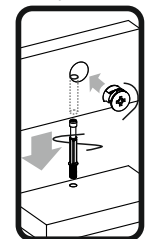
схема монтажа эксцентриковой стяжки
