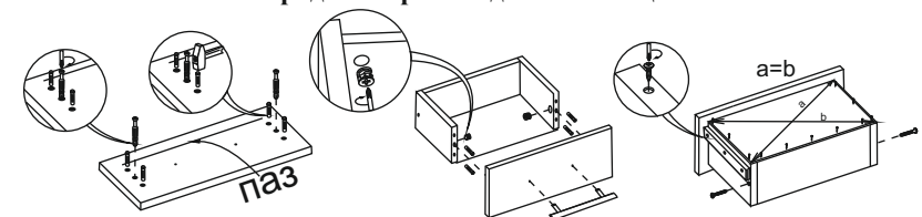
Порядок сборки выдвижного ящика
