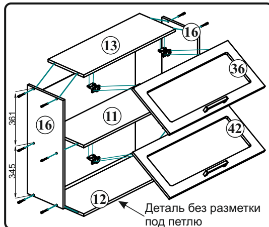
Схема сборки подвесного модуля
